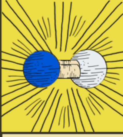
Kalcijum-oksid
