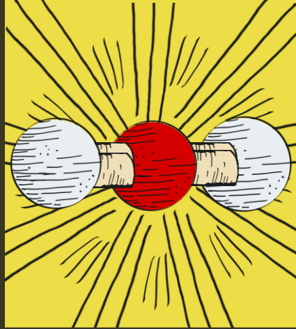
Ugljen-dioksid
